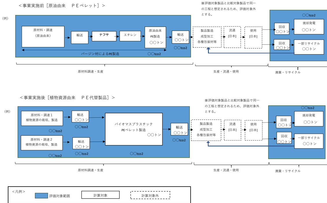
化石資源由来プラスチックを代替する再生可能資源由来素材の製造におけるライフサイクルフロー図（記載例）
